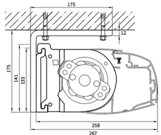
Plafondmontage
