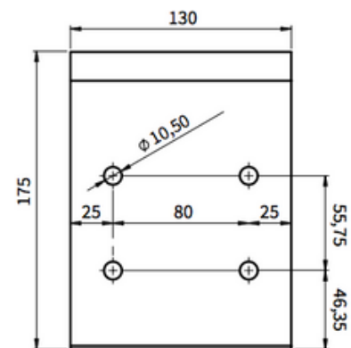
Vooraanzicht plafondsteun
